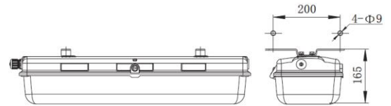
Deckenbefestigung
