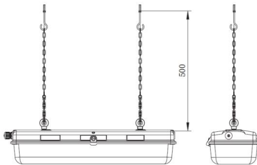
Kettenabhängung
