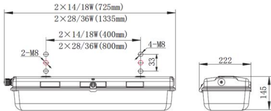
Abmessungen
